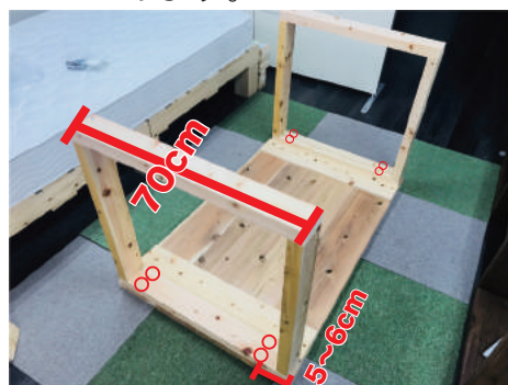
7 端から約5~6cmのところビス(65mm)で杉の板材に固定します。
